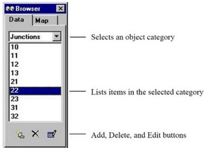
Fig. 5.2: Data browser.
