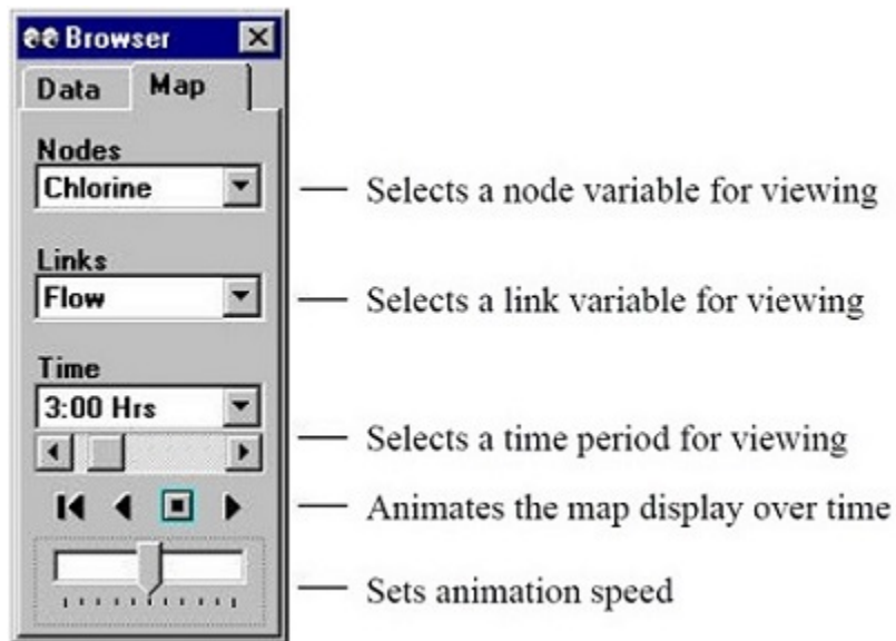
Fig. 5.3: Map browser.
